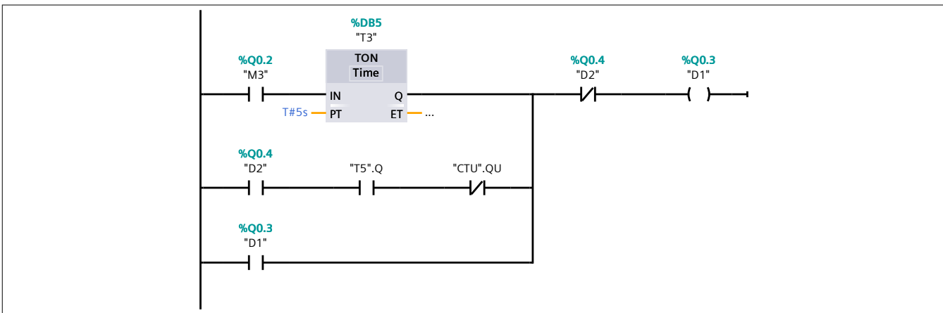
Network 5: D2
