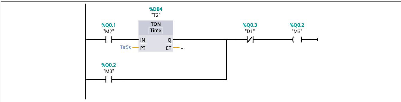
Network 4: D1
